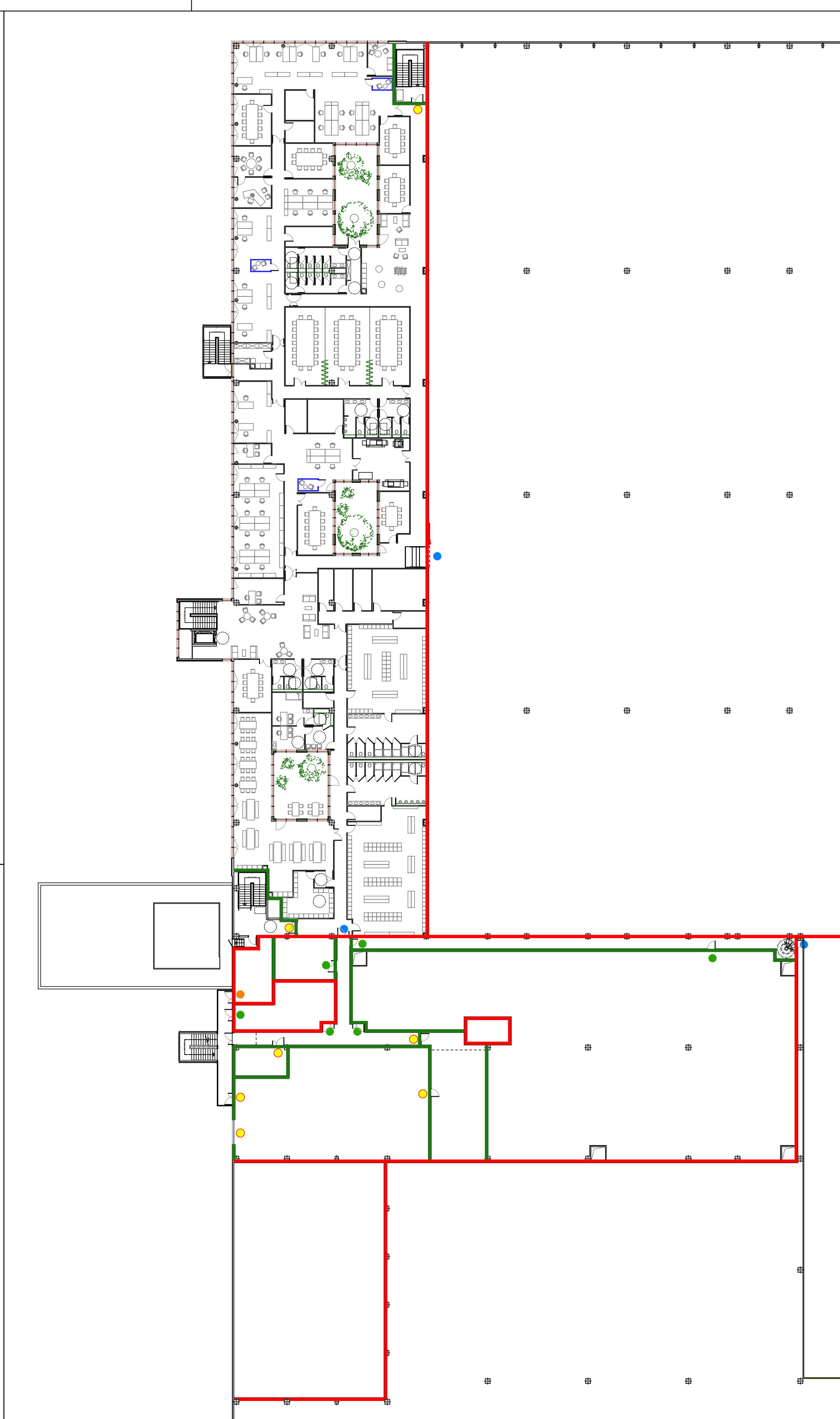
PLAN + 7.20. Bureaux et locaux techniques
