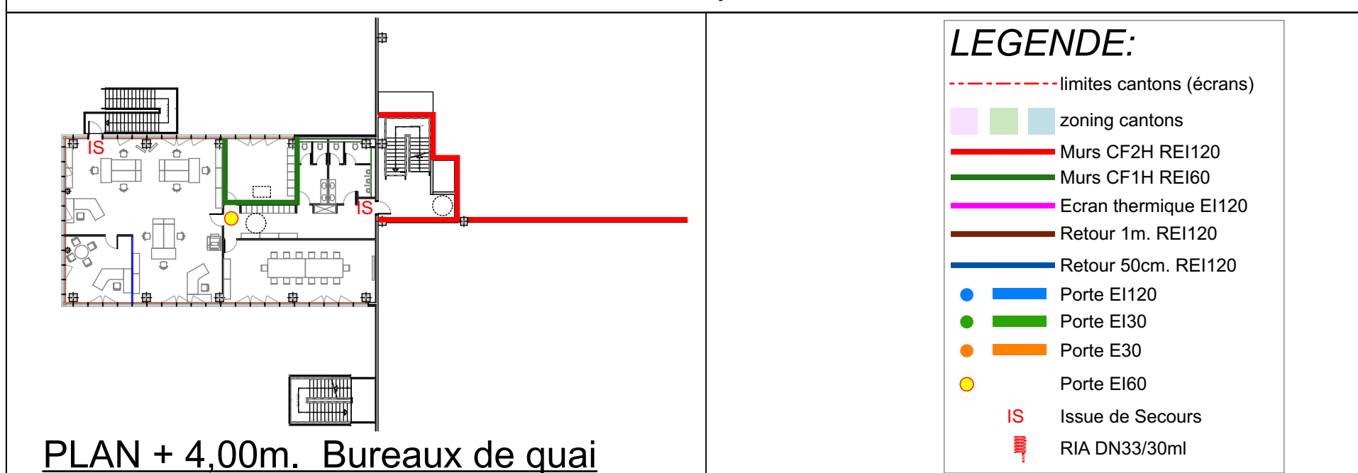
PLAN + 4.00m. Bureaux de quai
